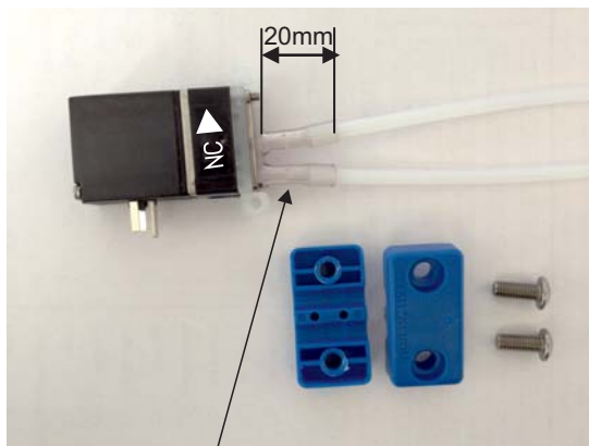
Verbindungsschlauch PVC, 5x3mm x 20mm lang, transparent
